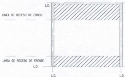
AMPLIACION PERMITIDA DESDE 8.00 M HASTA ALTURA MAXIMA 11.00 M
